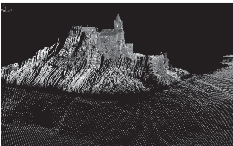
Figura 1 – Dati processati – Rilievo statico ad alta risoluzione 06, dinamico 08 e Batimetria
