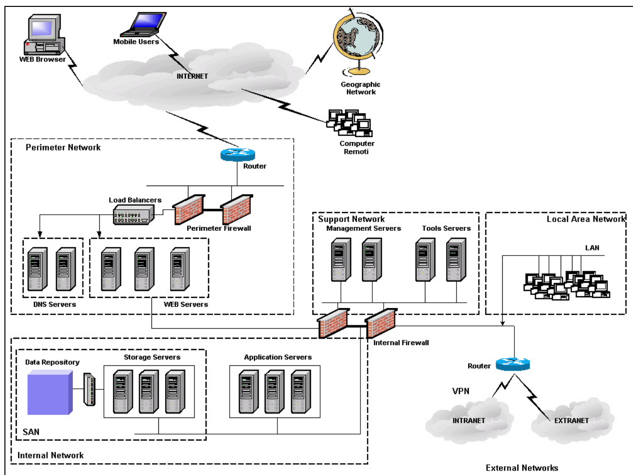
Figura 1 - Architettura di un'infrastruttura elaborativa operante in ambiente IDC
