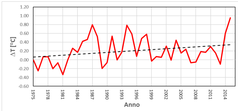
Figura 4. In rosso è mostrata la variazione della temperatura media annuale dell'area di studio rispetto al 1975 ( \Delta T ). In nero è riportata la linea di tendenza. (Fonte: Climatic Research Unit, University of East Anglia, http://www.cru.uea.ac.uk/data )
