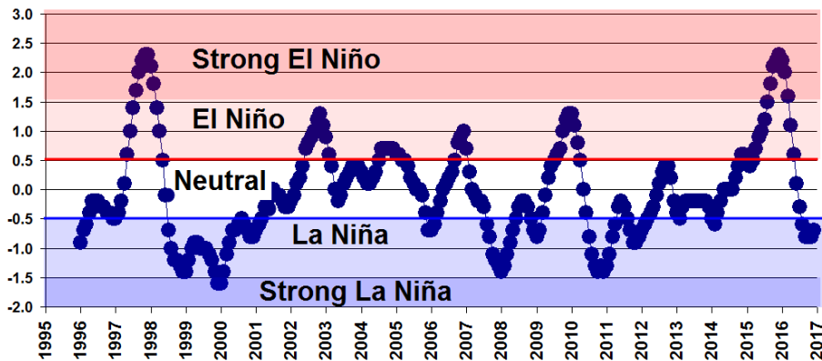
Figura 5. Serie temporali delle variazioni dell'indice CPC's Oceanic Niño Index (ONI) dal 1996 al 2017 (Fonte: Guam Hydrologic Survey, http://www.guamhydrologicsurvey.com/index.php/climate-and-weather/ )
