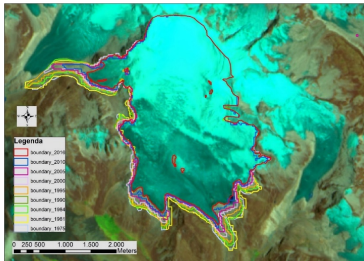
Figura 2. Variazione superficiale del ghiacciaio Chachacomani nel periodo 1975-2016 ricostruita mediante immagini satellitari Landsat e Sentinel-2.
