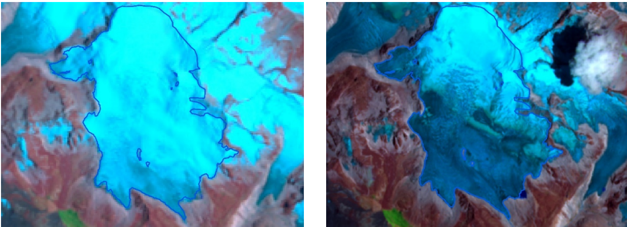
Figura 6. Esempio di stima dell'Accumulation Area Ratio. Pannello di sinistra: il ghiacciaio Chachacomani nel novembre 2011, stagione caratterizzata da La Niña. Si nota la superficie del ghiacciaio quasi interamente coperta da neve (AAR=0.73). Pannello di destra: il ghiacciaio Chachacomani nel novembre 2016, stagione caratterizzata da El Niño. La neve residua si trova praticamente solo sul plateau sommitale del ghiacciaio (AAR=0.37). Nell'immagine si nota il firn della stagione precedente.
