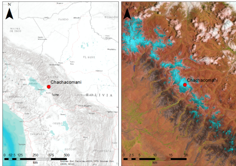
Figura 1. Pannello di sinistra: posizione del ghiacciaio Chachacomani rispetto alla città di La Paz. Pannello di destra: rappresentazione infrarosso falso colore della Cordillera Real (immagine Sentinel-2 del 13.11.2016).
