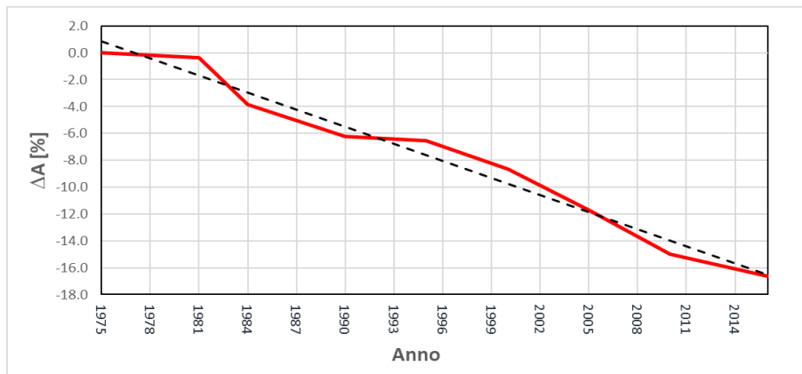
Figura 3. In rosso è mostrata la variazione superficiale del ghiacciaio Chachacomani rispetto alla copertura del 1975 ( \square A ). In nero è riportata linea di tendenza.
