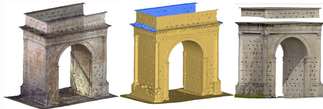
Figura 7 – Da sinistra: nuvola di punti dell'arco di Augusto acquisita con laser scanner, mesh dell'arco, mesh dell'arco texturizzata
